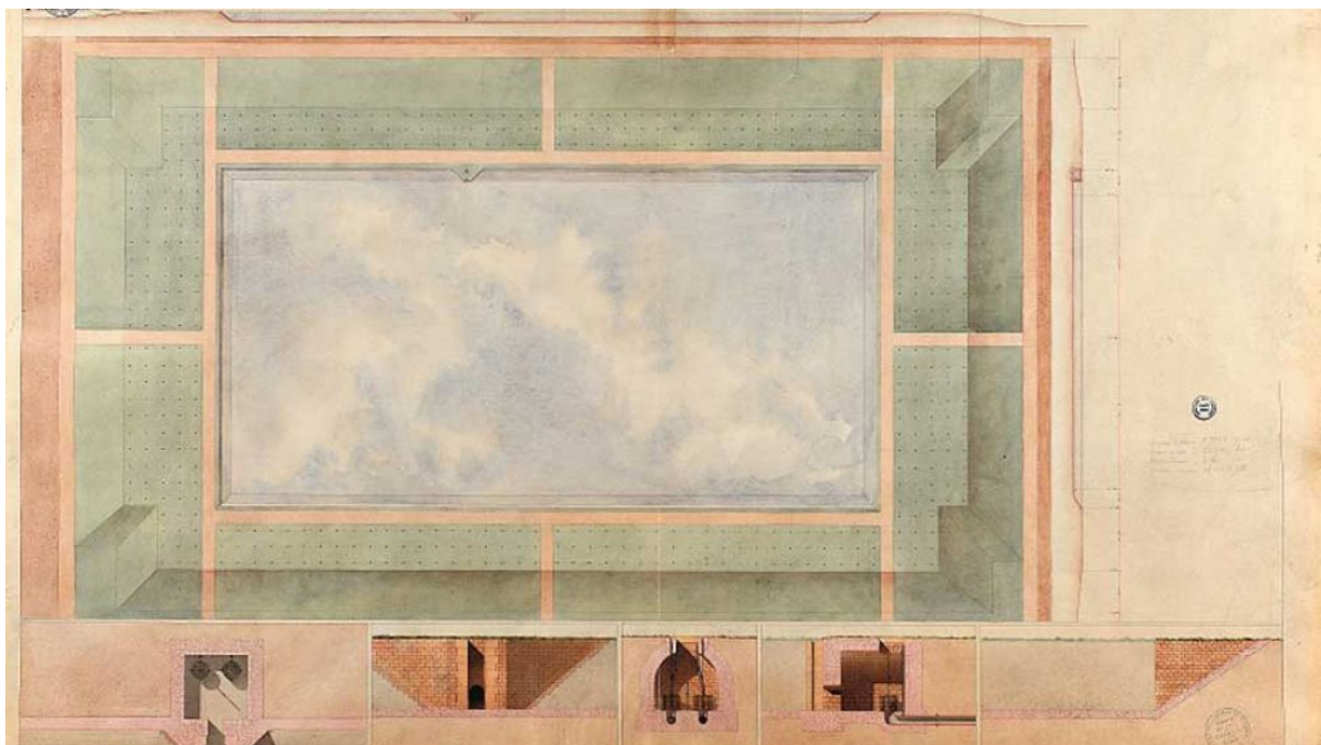
Projet de restauration du réservoir de Chèvreloup - 1 ère moitié du XIX e siècle
